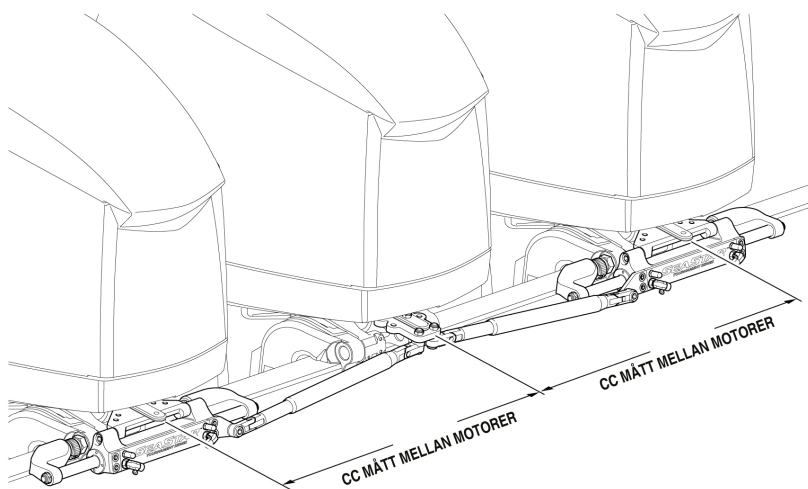
TRE MOTORER TVÅ CYLINDRAR
