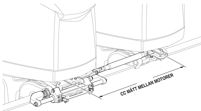
TVÅ MOTORER EN CYLINDER
